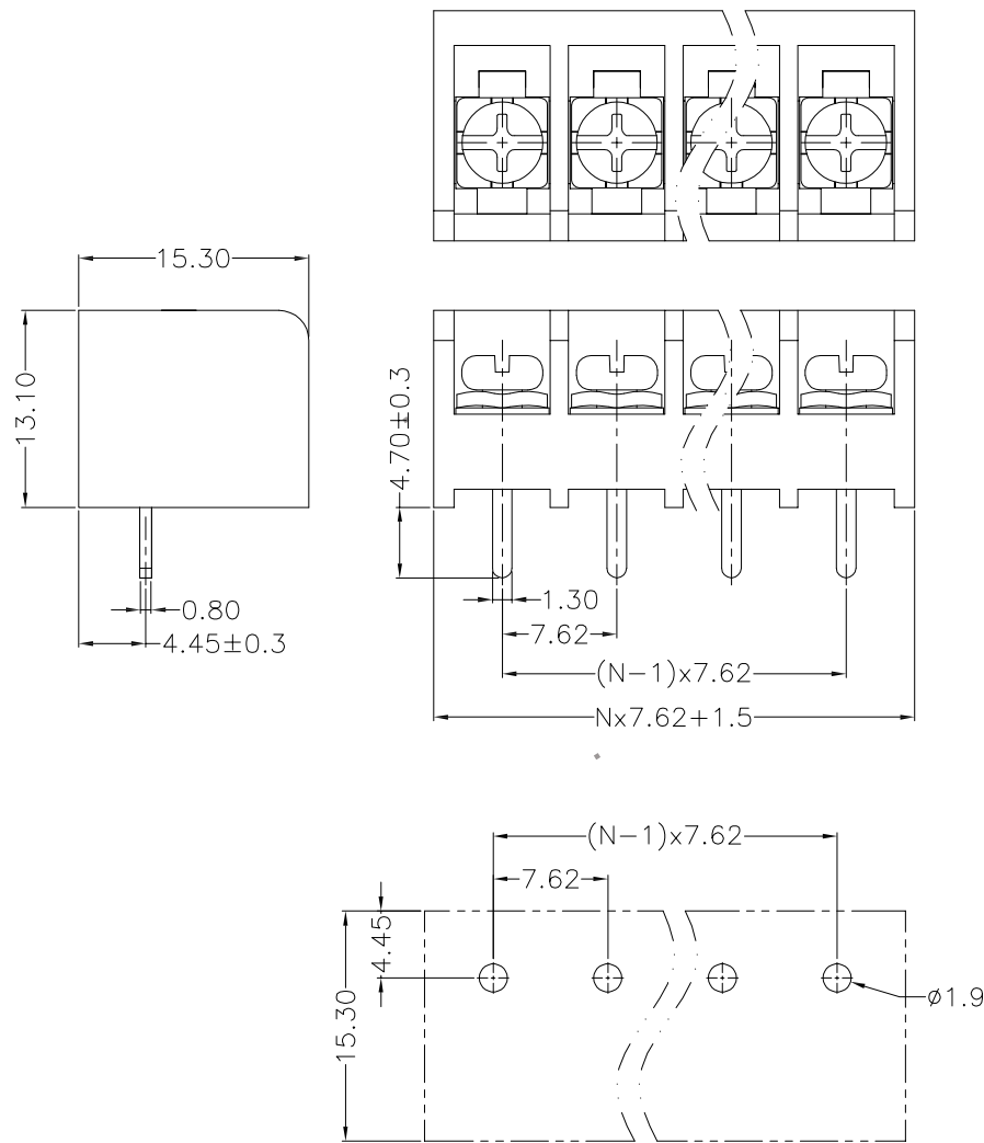
P.C.B.LAYOUT
