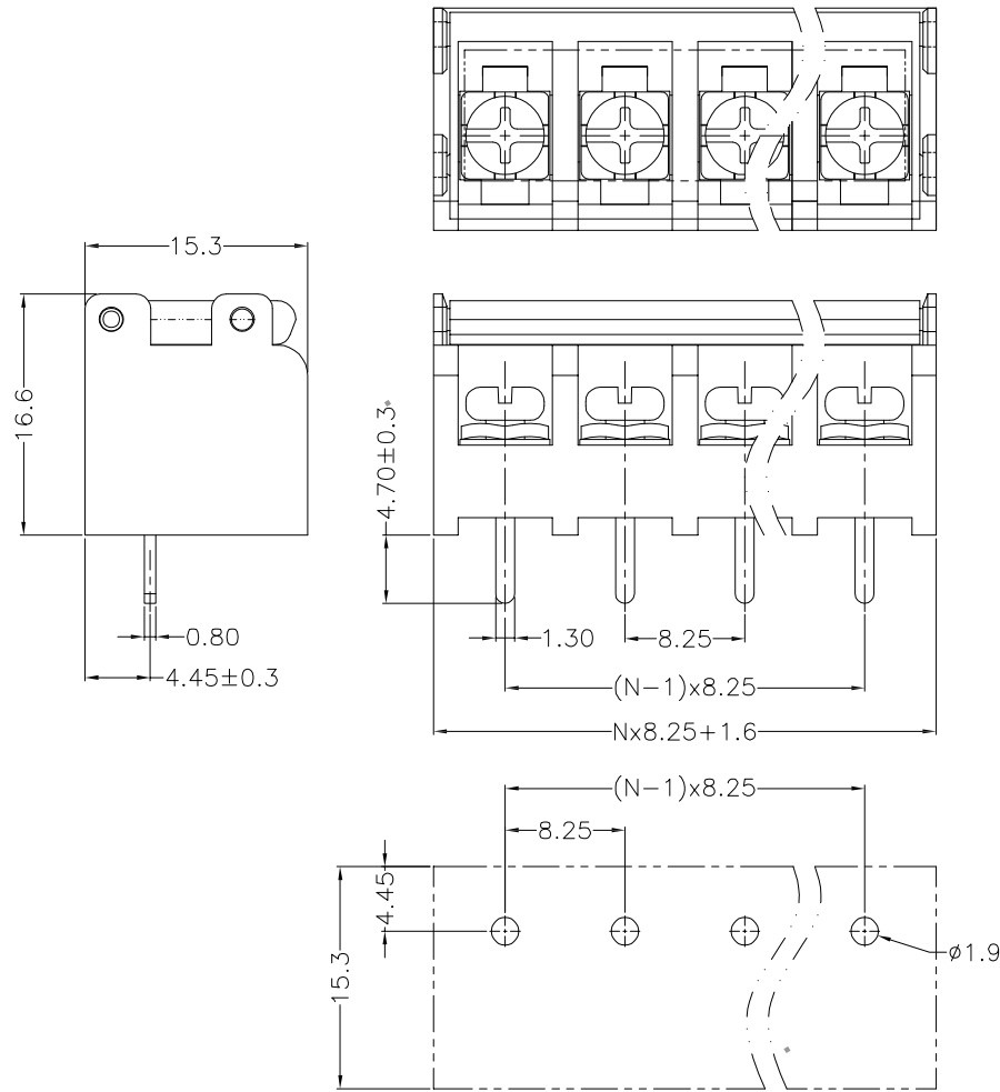
P.C.B.LAYOUT
